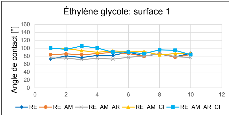
Figure-A II- 10 Variation d'angle de contact avec AM et sans facteur de rugosité avec l'éthylène glycol sur la surface rugueuse selon le nombre de répliques
