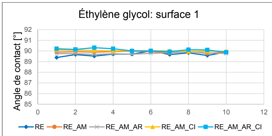
Figure-A II- 11 Variation d'angle de contact avec AM et avec facteur de rugosité avec l'éthylène glycol sur la surface rugueuse selon le nombre de répliques
