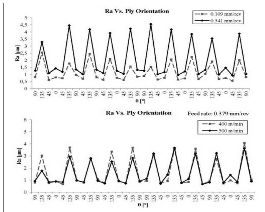
Figure 1.12 Variation de la rugosité de surface en fonction de l'orientation des fibres à vitesse d'avance et de coupe différente
