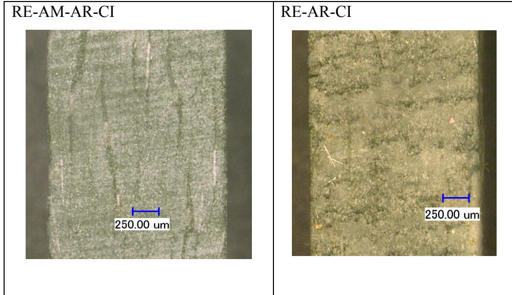
Figure 3.8 États de surface des différents stratifiés sur microscope (250 μm/div) (suite)
